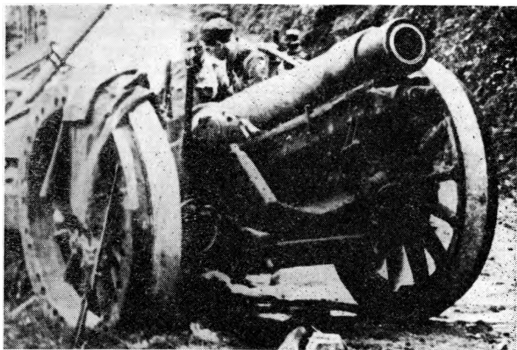
Težka havbica 149 mm M. 35, ki so jo partizani zaplenili Italijanom ob kapi- tulaciji in z njo obstreljevali Turjak
