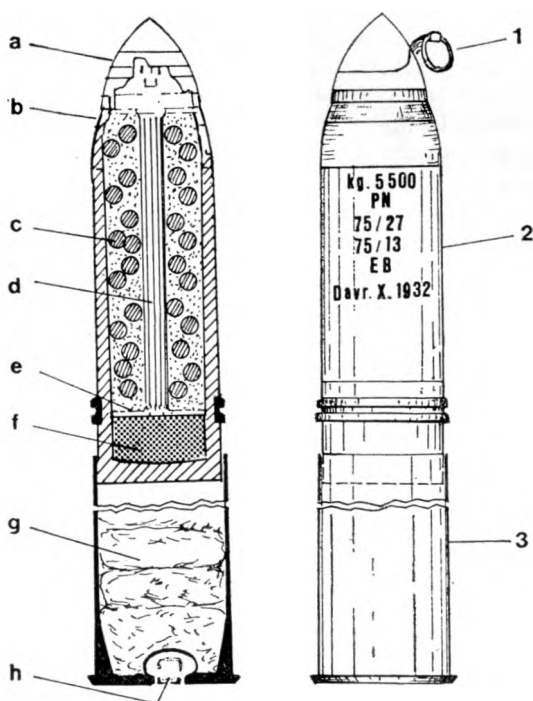
Šrapnel kal. 75 mm, zunanja podoba in v preseku
