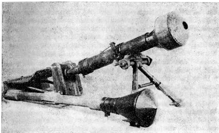
Partizanski top, imenovan partop
