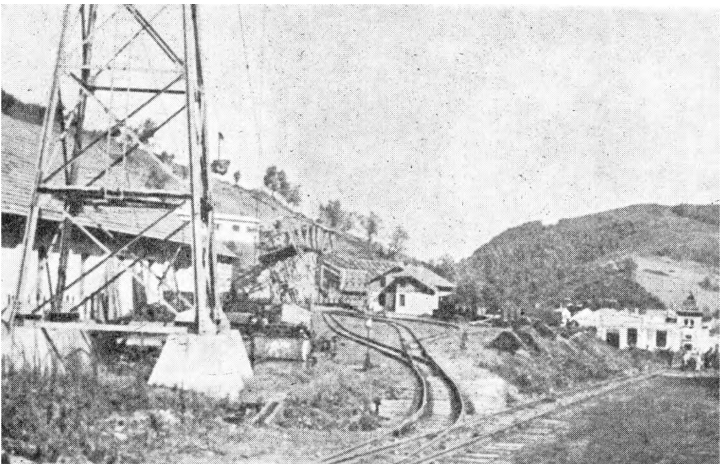
Žičara za izvlačenje rude u Ljubiji. Porušena 1942.
