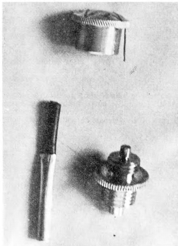
Dijelovi upaljača: kapica, eksplozivni dio i mehanički dio
